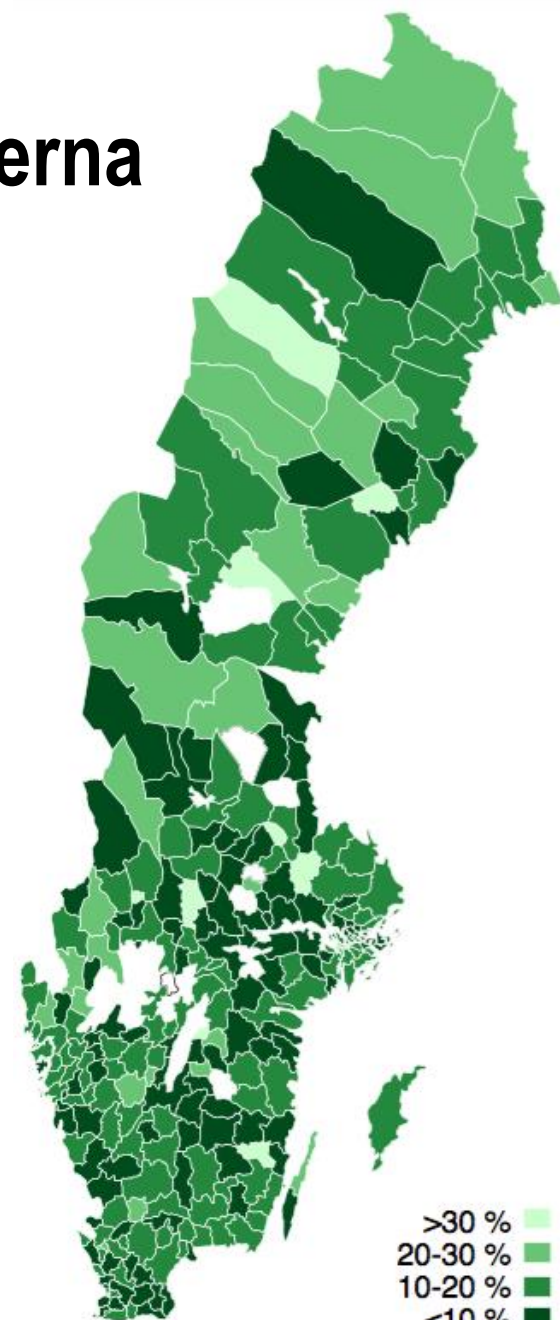
Procent ett anbud
