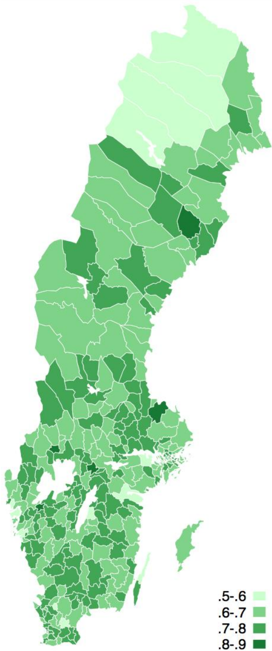
Institutionell kvalitet (KOLFU 2012)
